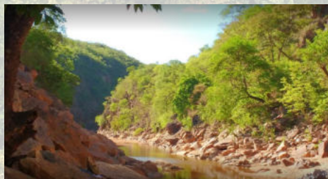
Figura 33 - Cânion Taboquinha
