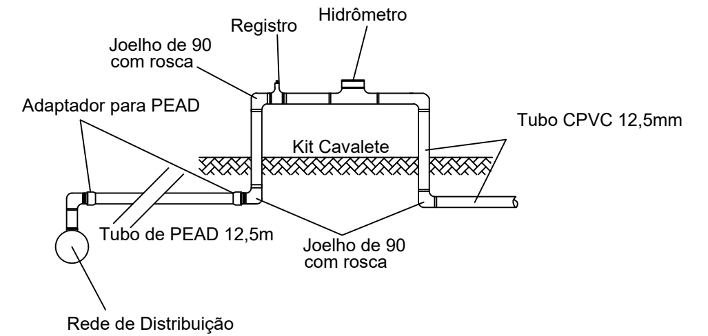
DETALHE DO RECEBIMENTO DE ÁGUA S/Escala
