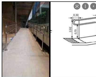
DET. RAMPA sem esca
